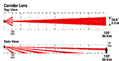
EC301D karakterisztika
